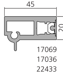
Stützenprofil links / rechts Support profile left / right
