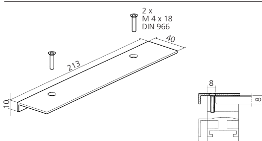
Deckleiste – End, Aluminium mit Seitenschutz Covering profile – end with side protection
